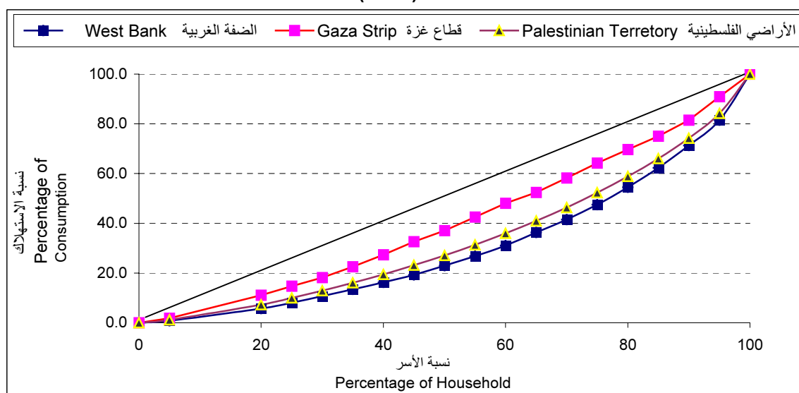
جدول 42.2 (تابع): منحنى لورنس Table 2.42 (Cont): Lorenz Curve
