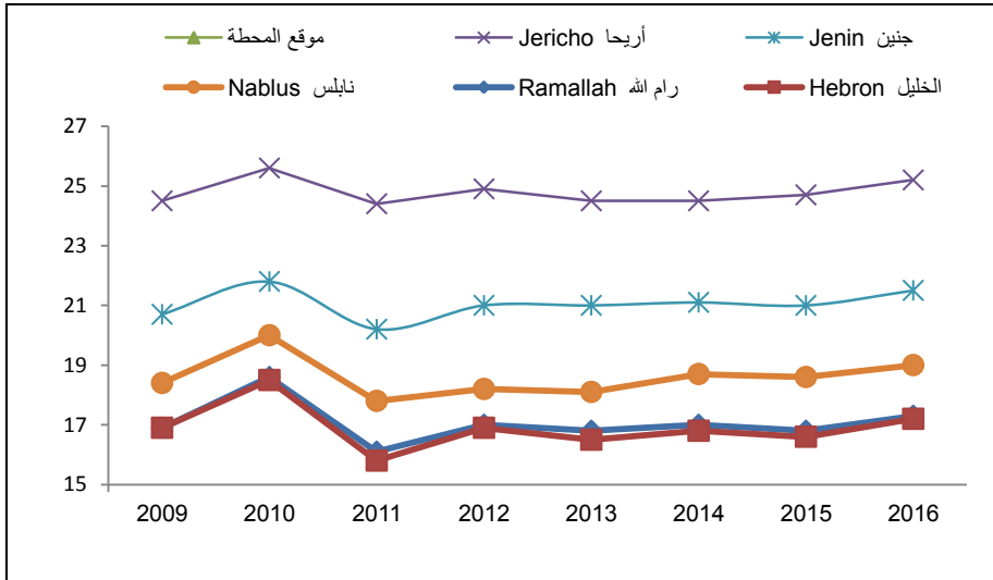
المعدل العام لحرارة الهواء (م) فف فلسطين حسب السنة وموقع المحطة، 2016-2009 Mean of Air Temperature (C°) in Palestine by Year and Station Location, 2009-2016
